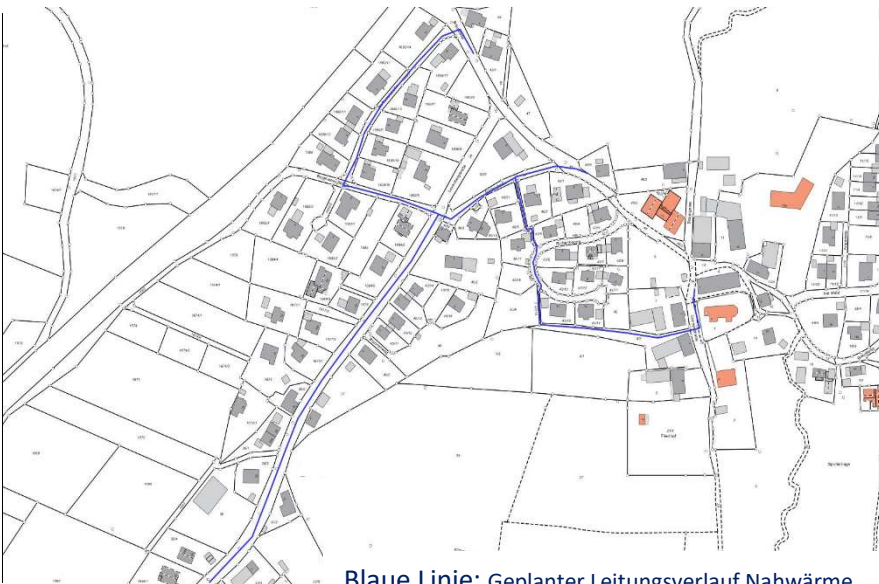
Blau e Linie: Geplanter Leitungsverlauf Nahwärme
